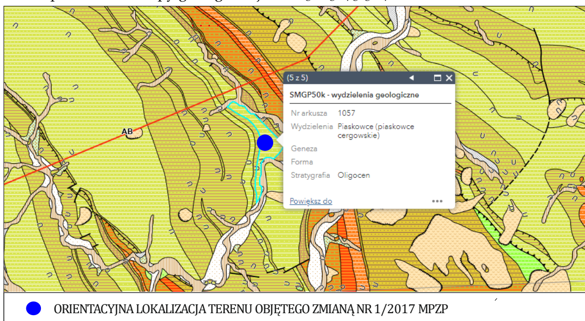
Ryc. 5. Orientacyjne położenie terenu objętego sporządzeniem Zmiany Nr 1/2017 MPZP Piaskowców Cergowskich Komańcza – Jawornik Gmina Komańcza, Województwo Podkarpackie na tle mapy geologicznej. Źródło: geologia.pgi.gov.pl
