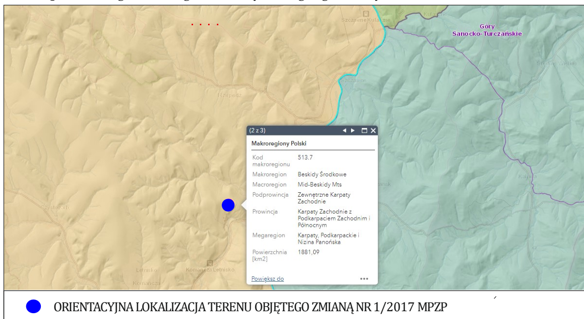
Ryc. 4. Orientacyjne położenie terenu objętego sporządzeniem Zmiany Nr 1/2017 MPZP Piaskowców Cergowskich Komańcza – Jawornik Gmina Komańcza, Województwo Podkarpackie względem regionów fizyczno-geograficznych. Źródło: geologia.pgi.gov.pl
